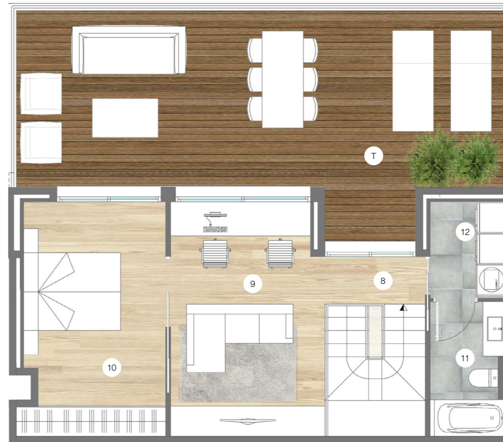
PLANTA SOTACOBERTA
